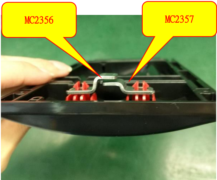
图四，装入 MC2356 在 PM2638 上，MC2356 朝中间
