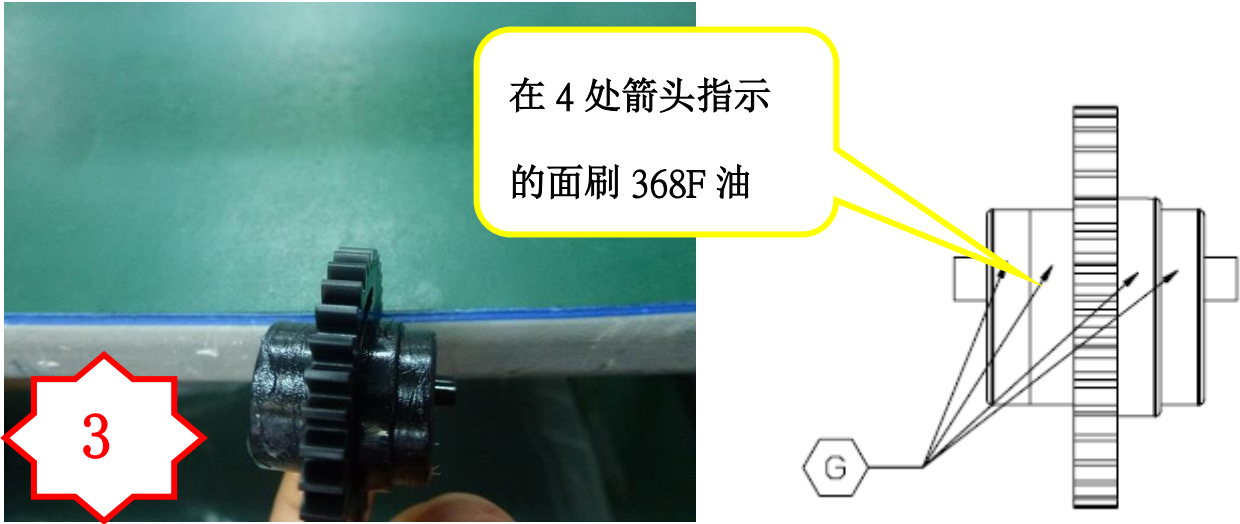
图三，在 4 处箭头指示位置刷 368F 油
