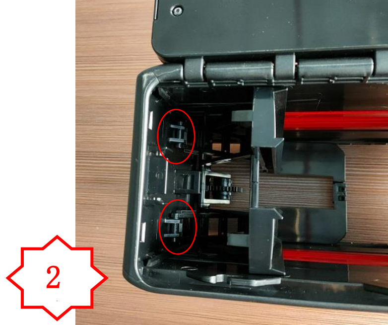
图二，装入起落架，红色圈位置需卡到位
