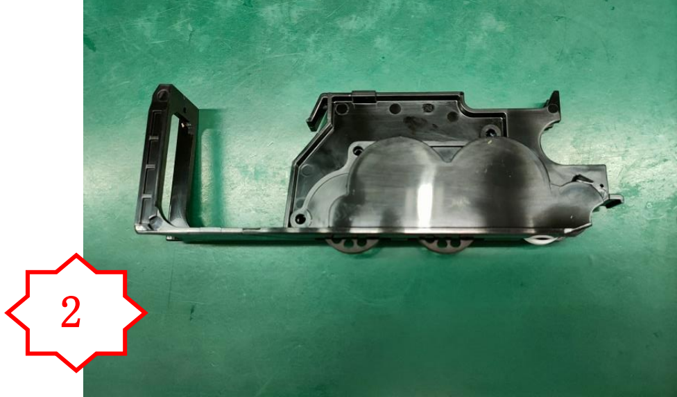
图二,将 PM694 盖在 PM2934-1 上
