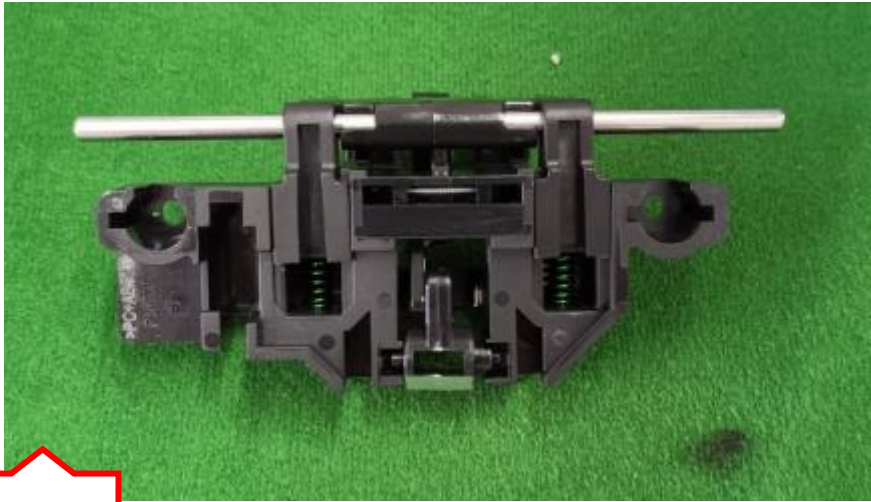
图三, 将 MC259 穿过两个 PM690 和 PM2022 的孔内
