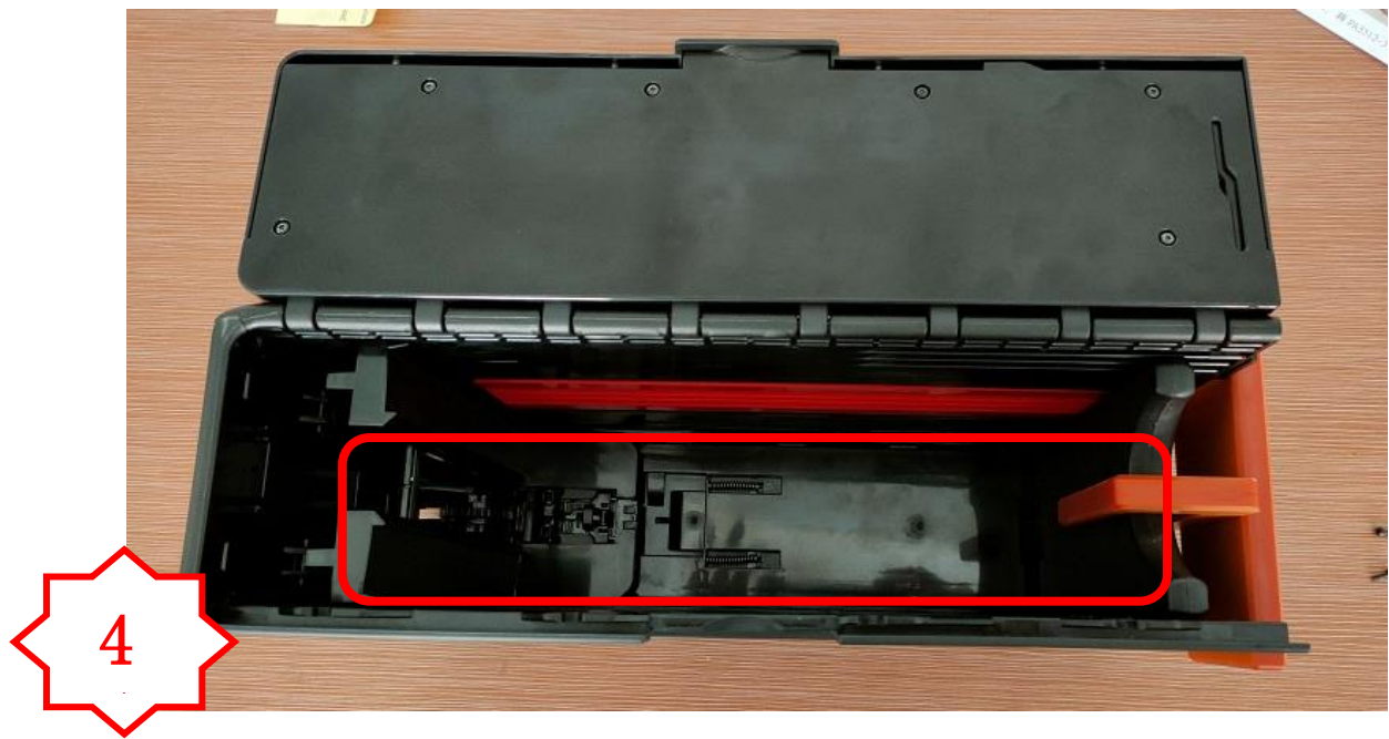
图四，装入一个 PA3312-3 在 PA3110-3 下方
