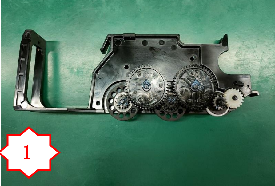
图一，在 6 个柱子顶部及齿轮顶部刷适量 368F
