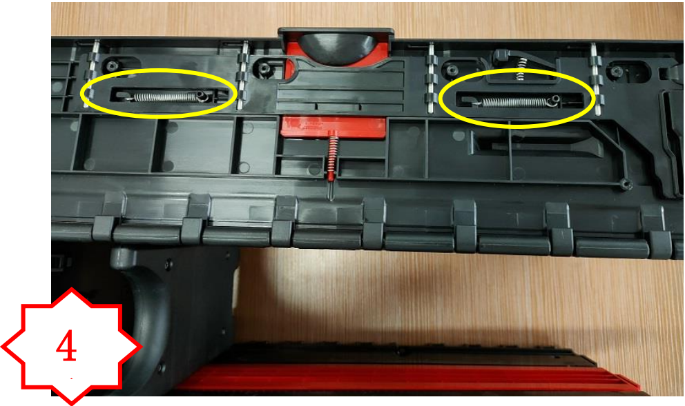
图四，装入 2 个 SP176
