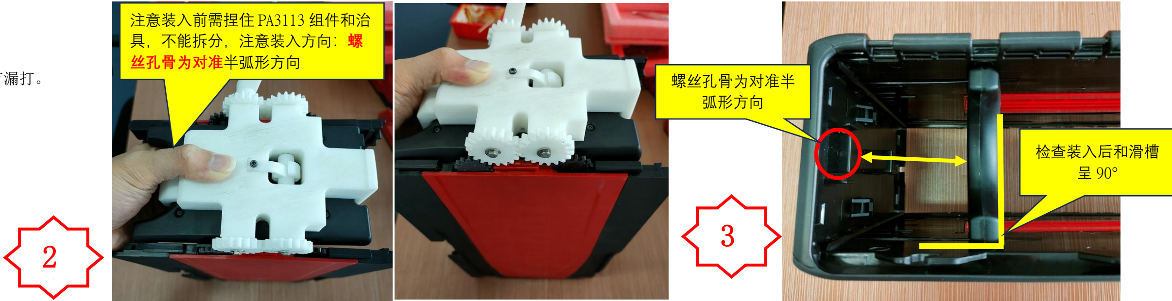
图三，检查 PA3113 组件装入后和滑槽呈 90°，当将 PA3113 组件往外推时需顺畅复位。
