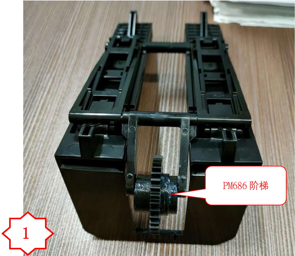
图一，装入 1 个 PM686，有阶梯的一侧朝右装入 PM687
