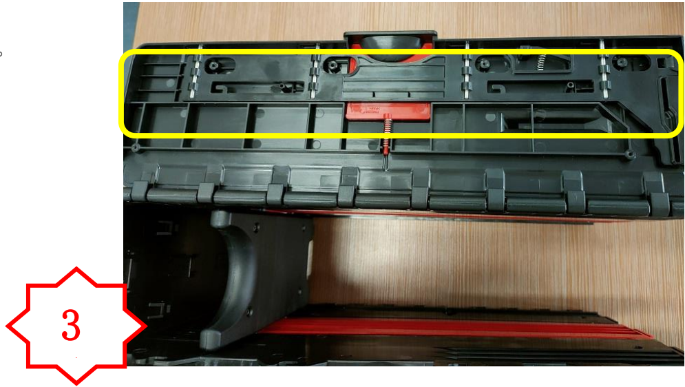
图三，将 PA3110-1 装到组件上
