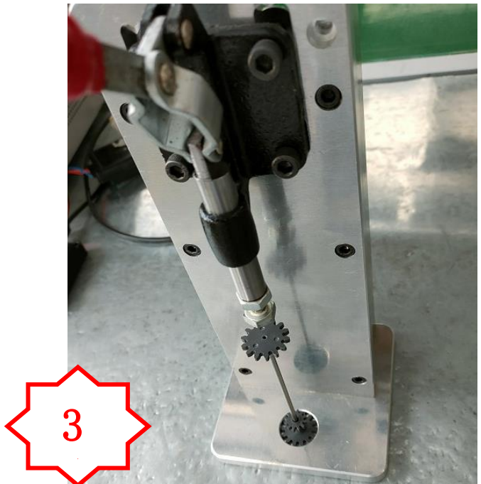
图三，在 MC2385 另一侧装入 PM2895，然后放到治具上压合
