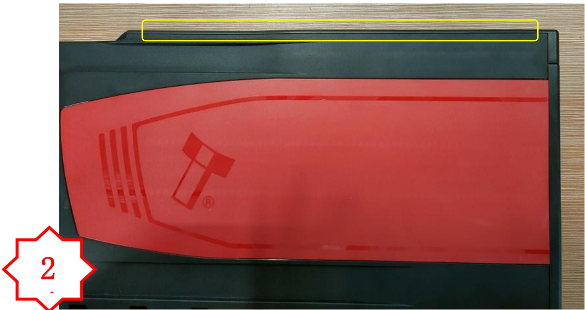
图二，打完螺丝后检查打螺丝固定的两侧是否有超过 0.4 的间隙
