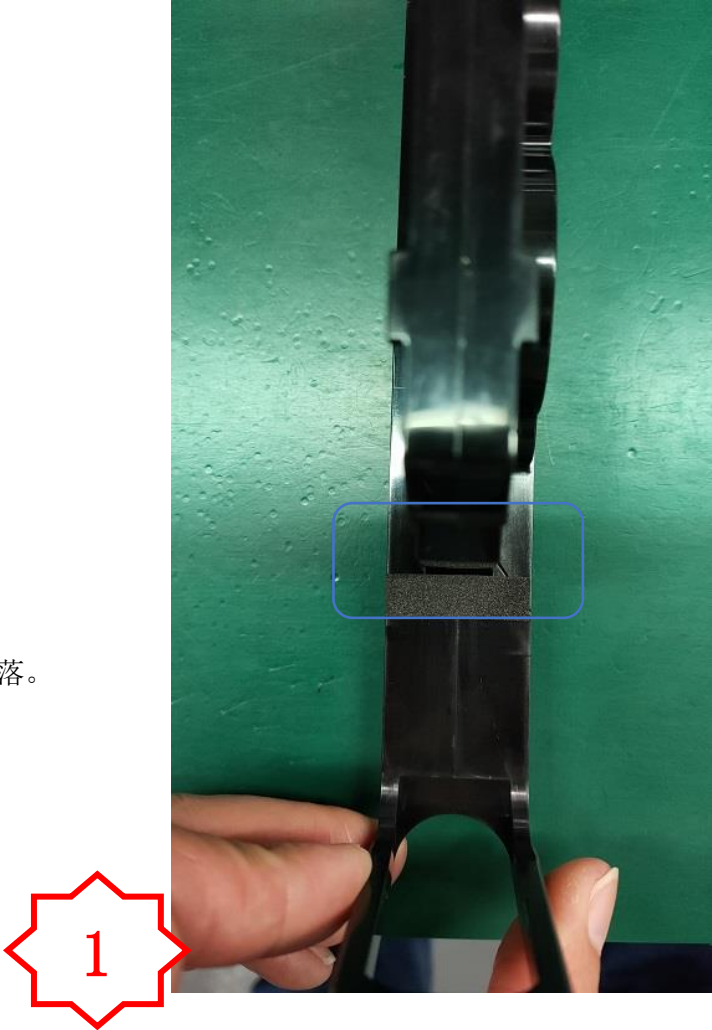
图一，在 PM693 组件上贴 LB2104，两侧不高 于塑料平面，顶部贴平
