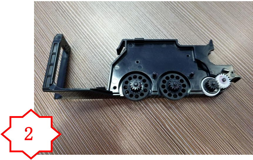
图二，将两个 PM634+FD115，一个 PM635 装入 PM693
