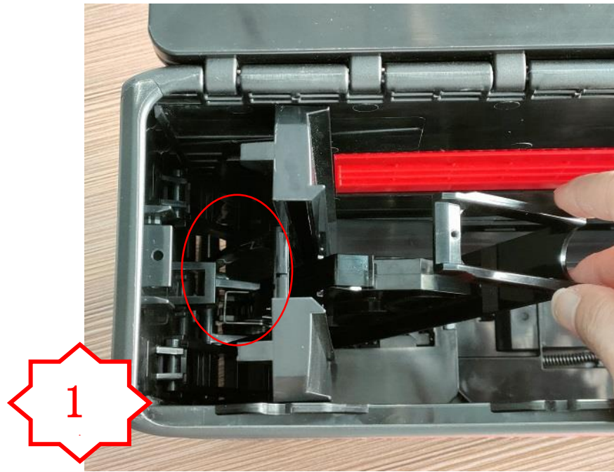
图一，将 PA2924 组件对准起落架上的 PM686 装入
