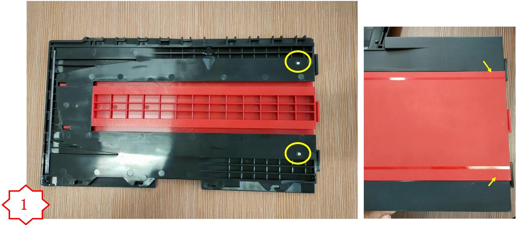
图一，打入 2 个 SC128，螺丝打到位后 PM2880 表面不能有顶白
