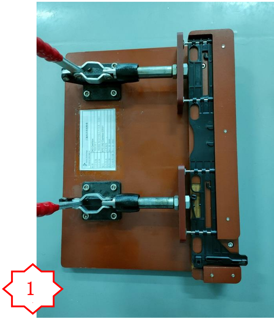
图一，用治具将 4 个 MC2379 压到 PM2888 的孔，轴压到底后外漏尺寸为 7.0±0.1（4 个位置）
