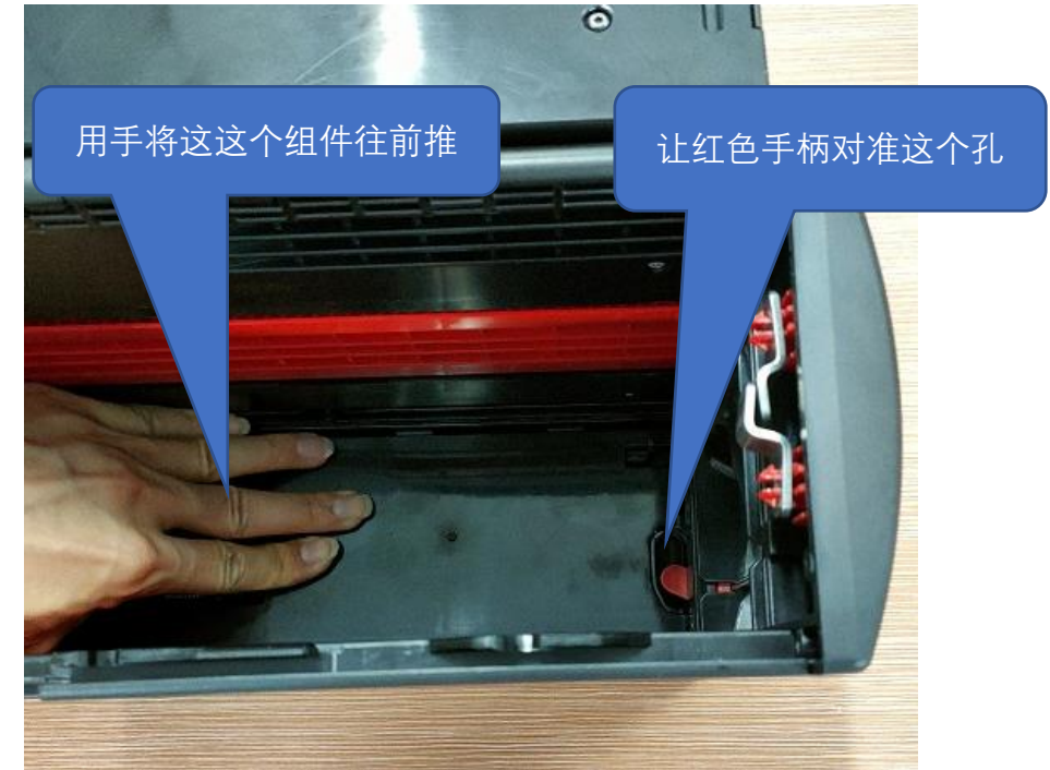
图一，将 PA3309-3 装到口部然后往下面推，然后将底部的组件孔对准红色手柄
