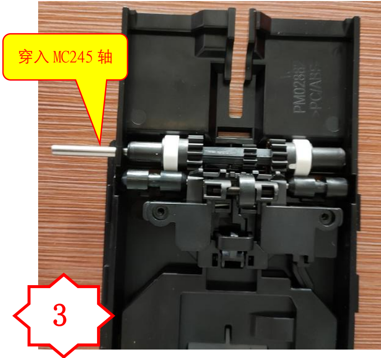
图三, 将 MC245 压进孔里
