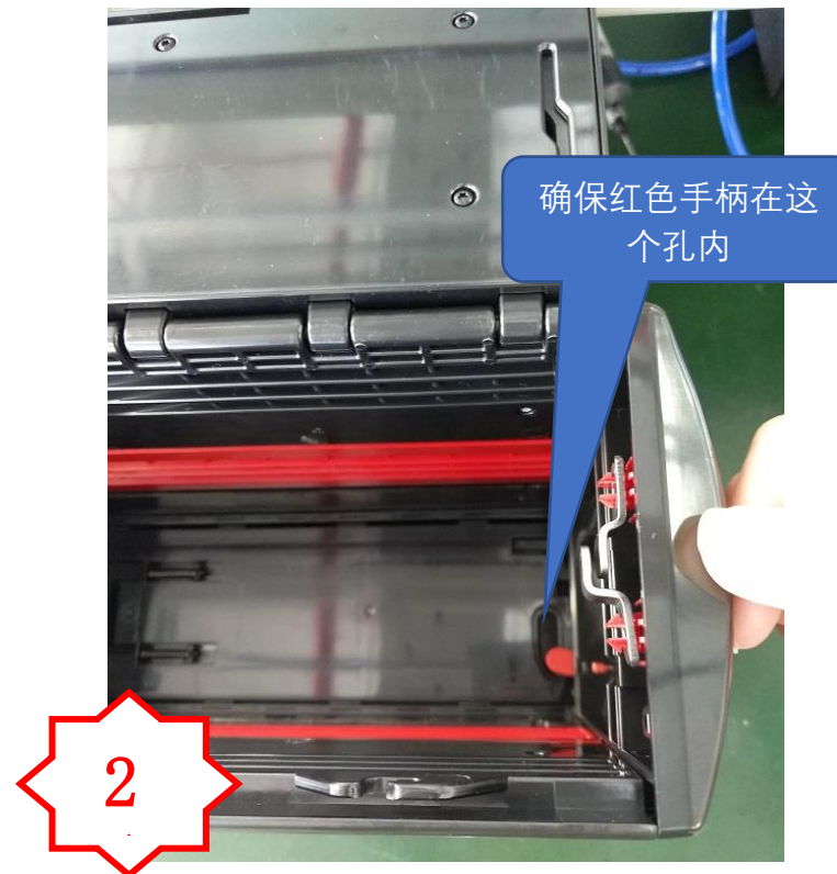
图二，将组件完全推到底
