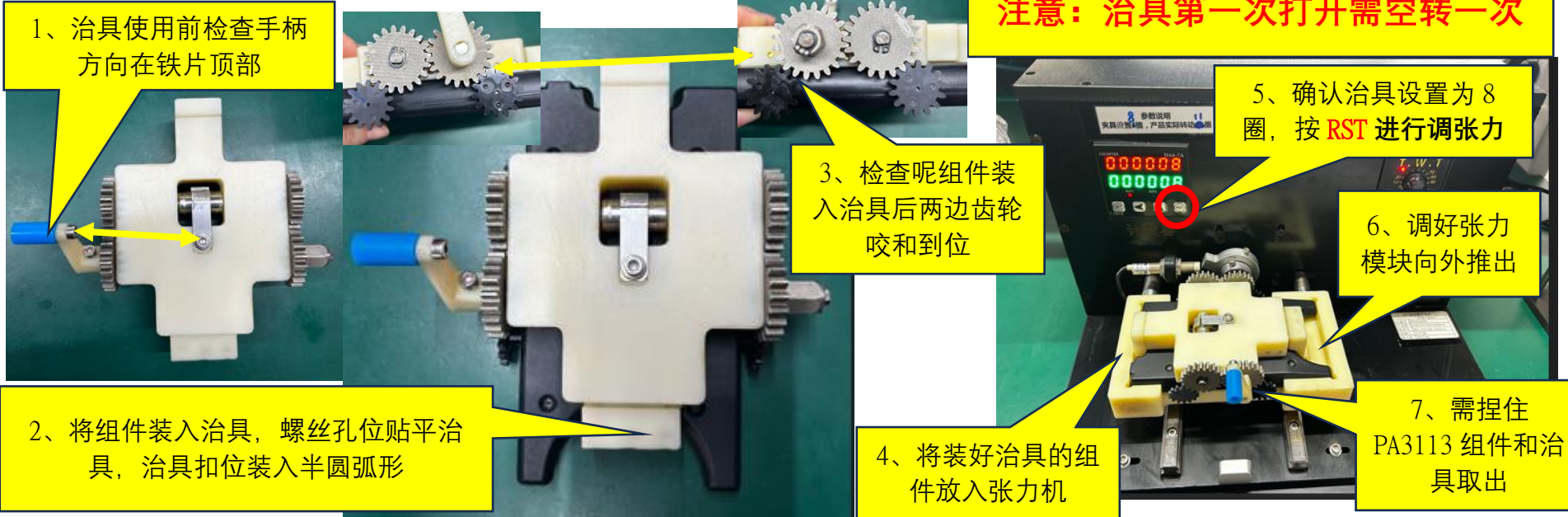
图一，治具设定为 8 圈，将 PA3113 装到治具上，按图示要求进行调张力，完成后，实物检查为 11 圈，需生产前检查 1PCS 后再批量生产。
