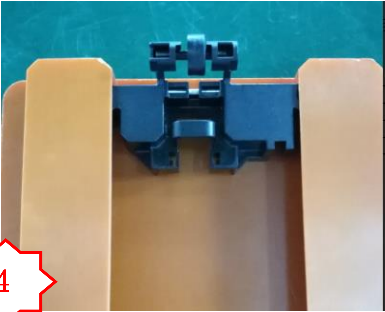
图二,将 PA3111-1 放入治具中
