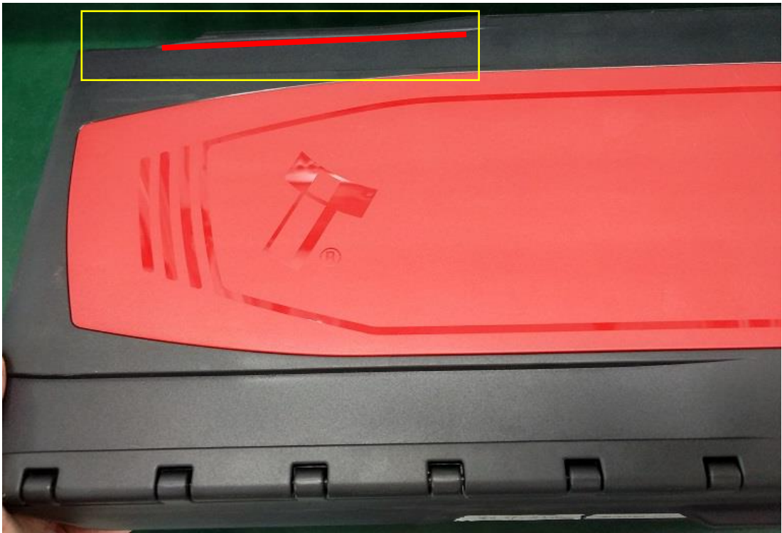
3 · 在内箱如图所示的黄色区域内用抹有油脂的海绵进行擦拭，确保红色线位置都要擦拭到位。
