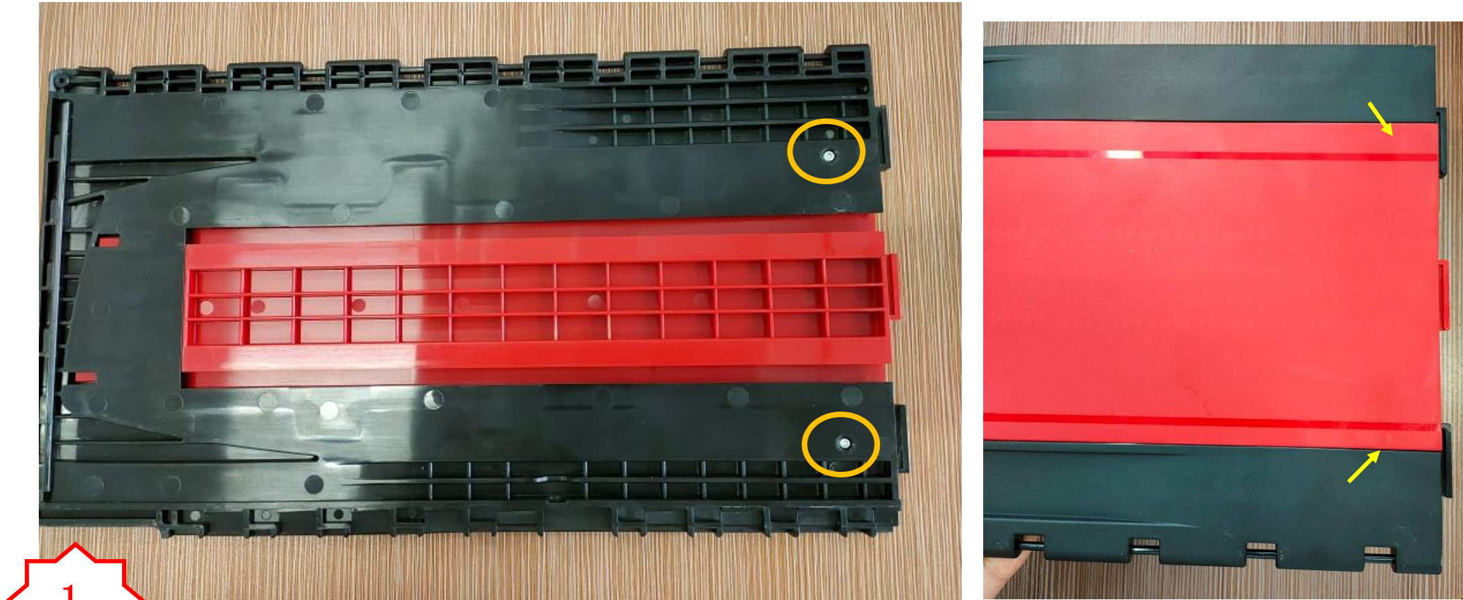
图一，打入 2 颗 SC128，PM2881 表面不能顶白
