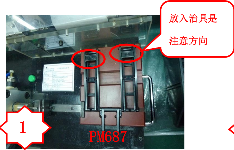
图一,将两个 PA3112-2 和 PM687 装入治具中
